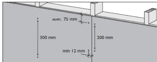
Наиболее важные размеры креплений
